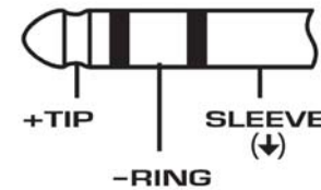
PINAGEM DO PLUG STEREO P10 (1/4" TRS)
