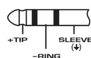
PINAGEM DO PLUG STEREO P10 (1/4"TRS)
