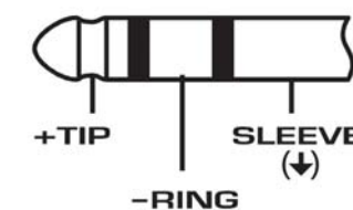
PINAGEM DO PLUG STEREO P10 (1/4"TRS)
